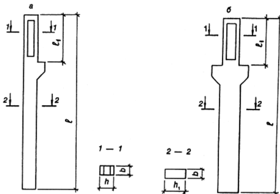
a - колонна для крайних рядов; б - колонна для средних рядов Черт.3
