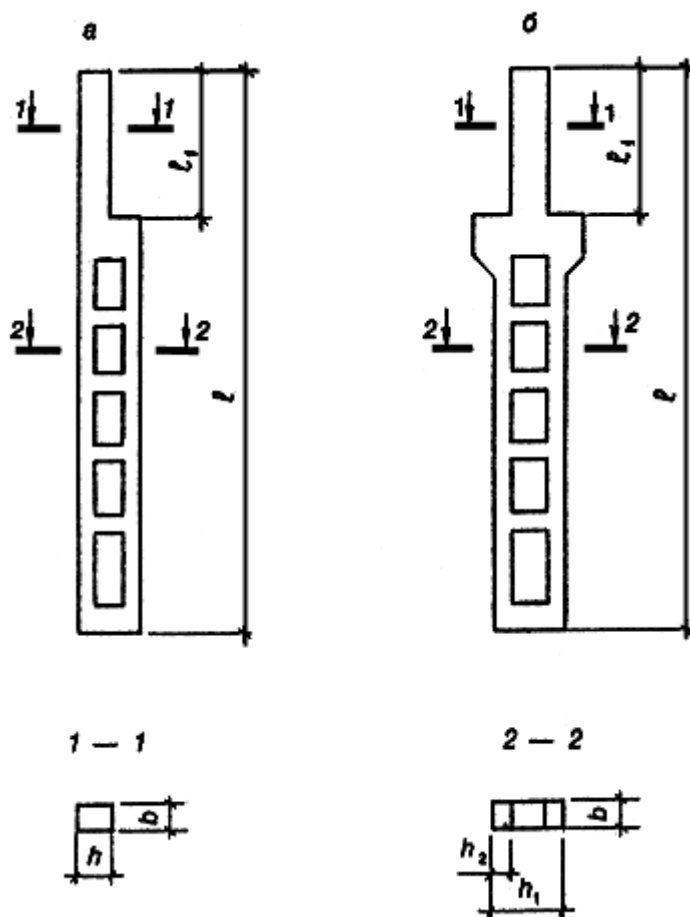
a - колонна крайних рядов; б - колонна средних рядов Черт.6
